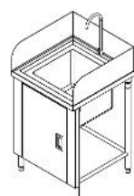
M8 อ่างล้างล้าง
