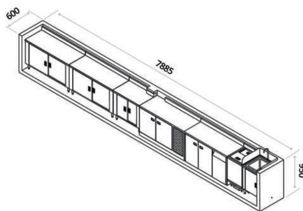
M3 ตู้เคาน์เตอร์สแตนเลส
