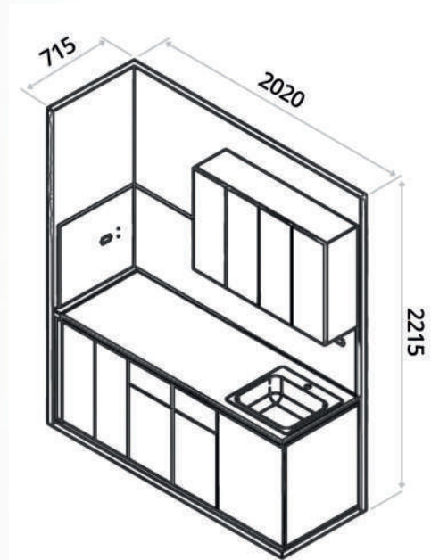
M3 ชั้นวางเครื่องปรุง
